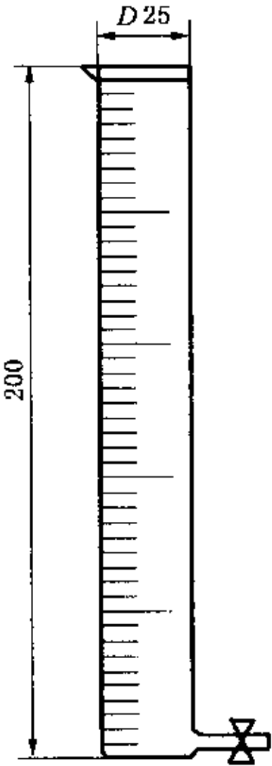
图 6 玻璃透视管
