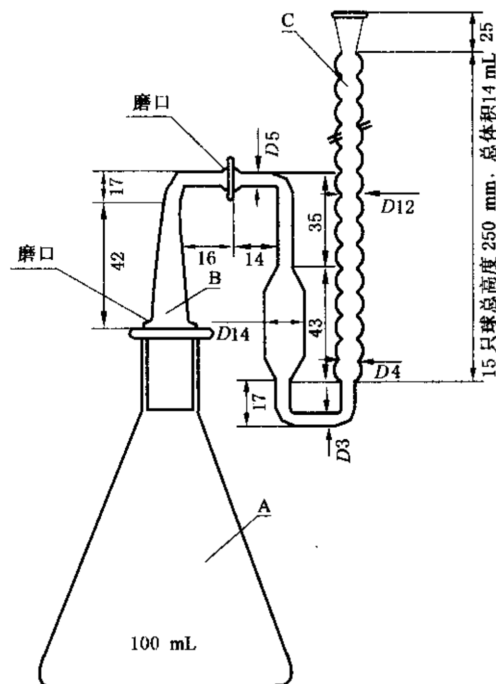
图 3 定砷仪
