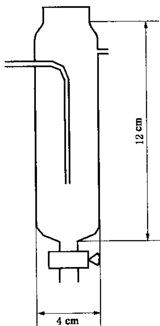
图 5 洗气瓶
