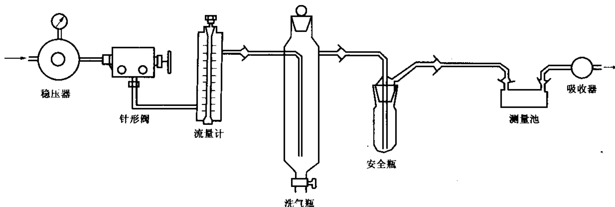
图 4 吹气(或吸气)测定系统装置
