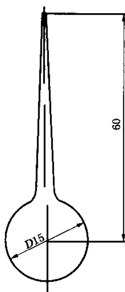
图 1 安瓿球
