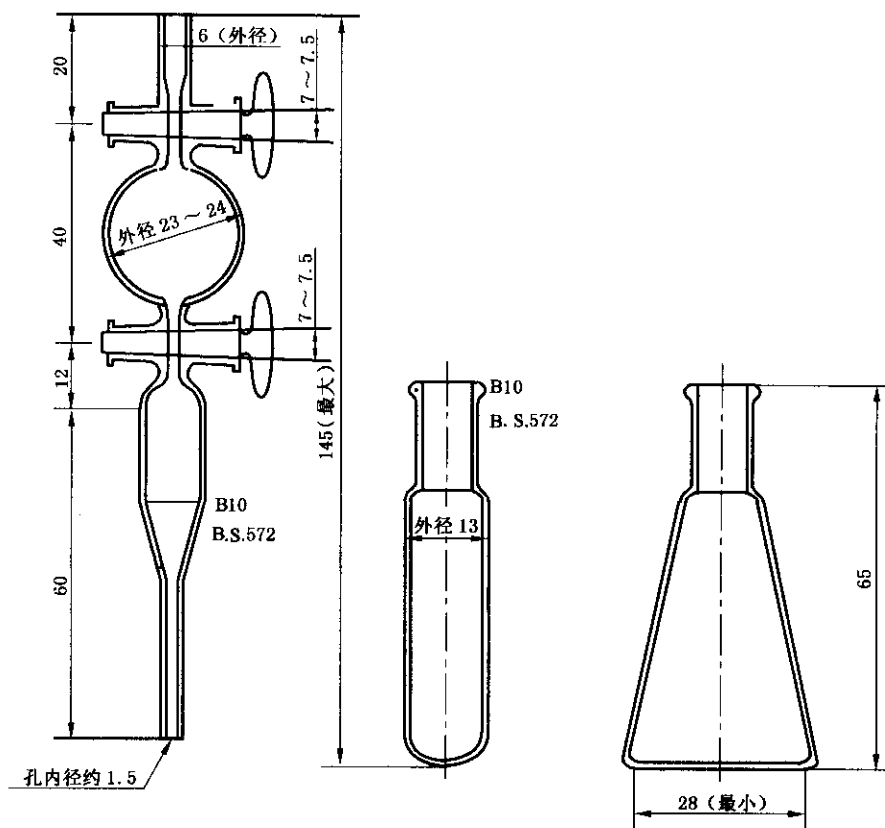
图 2 称量移液管
